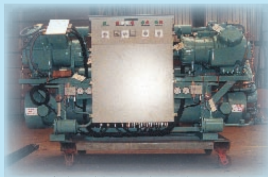
Refroidisseur de liquide (250 kW - Condensation eau de mer)
